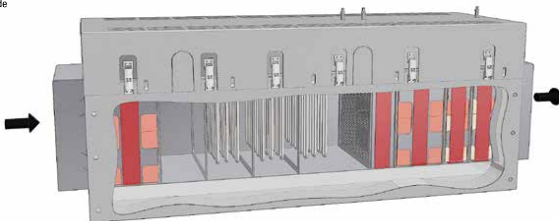
Représentation schématique d'une postcombustion catalytique (KNV)
