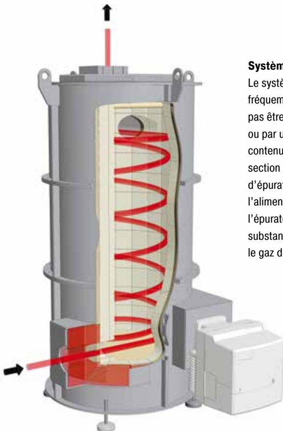
Représentation Schématique d'une postcombustion thermique (TNV)
