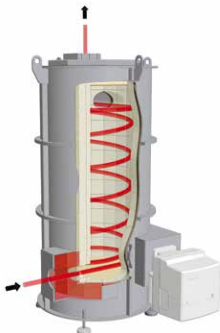
Représentation Schématique d'une postcombustion thermique (TNV)
